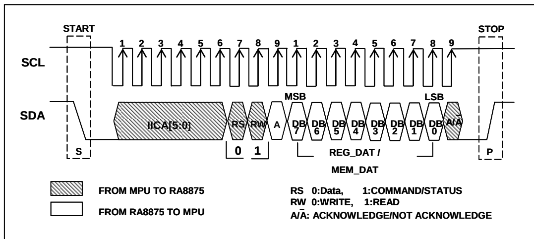
图 6-23 : IIC 数据总线的数据读取
