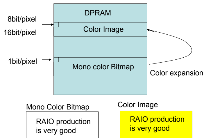
图 7-63 : BTE 移动搭配颜色扩充功能数据转换示意图
