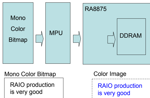
图 7-61 : 通透性颜色扩充功能数据区块图
