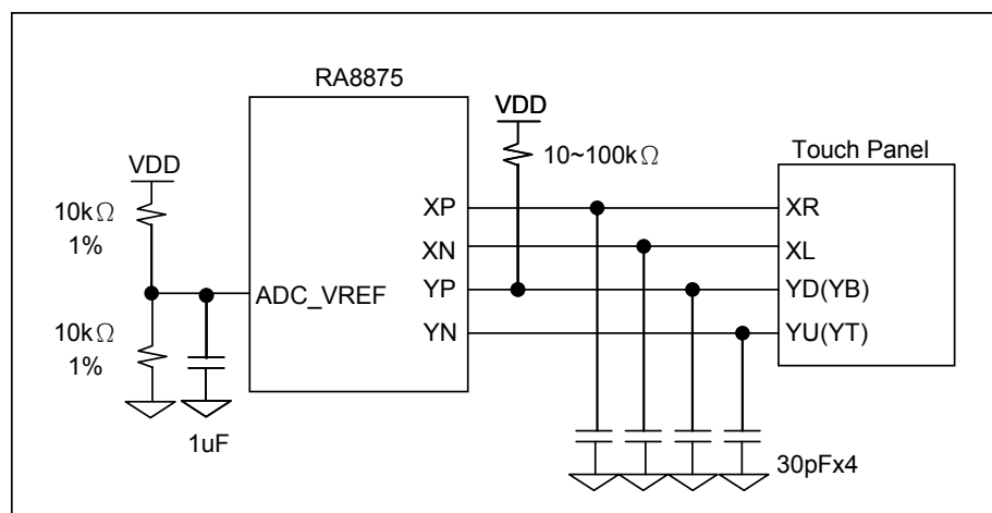
图 6-48 : 4-wire 触控面板应用电路
