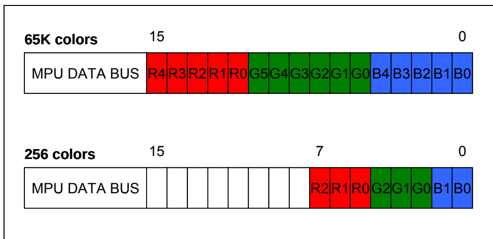
图 6-33 : MCU 16-bit 时 Data Bus 所对应到的 RGB 数据
