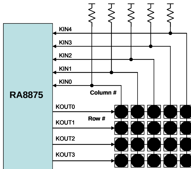
图 6-49 : 4x5 键盘的基本应用电路
