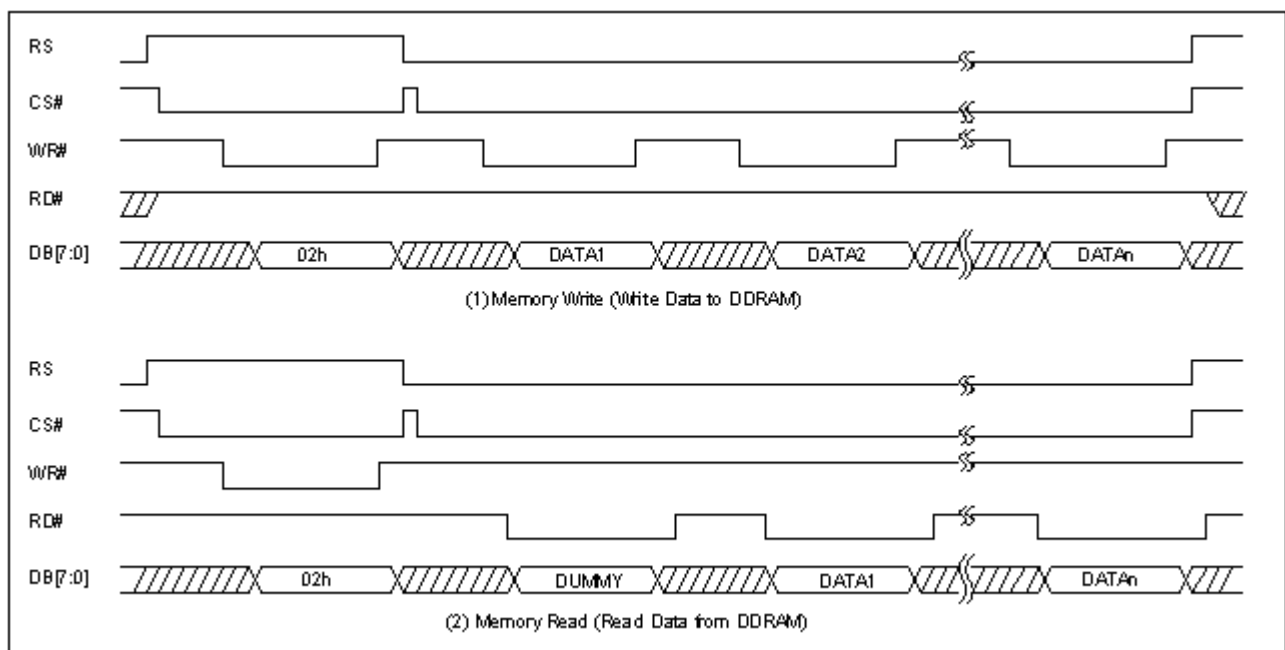
图 6-30 : 8080 内存写入与内存读取
