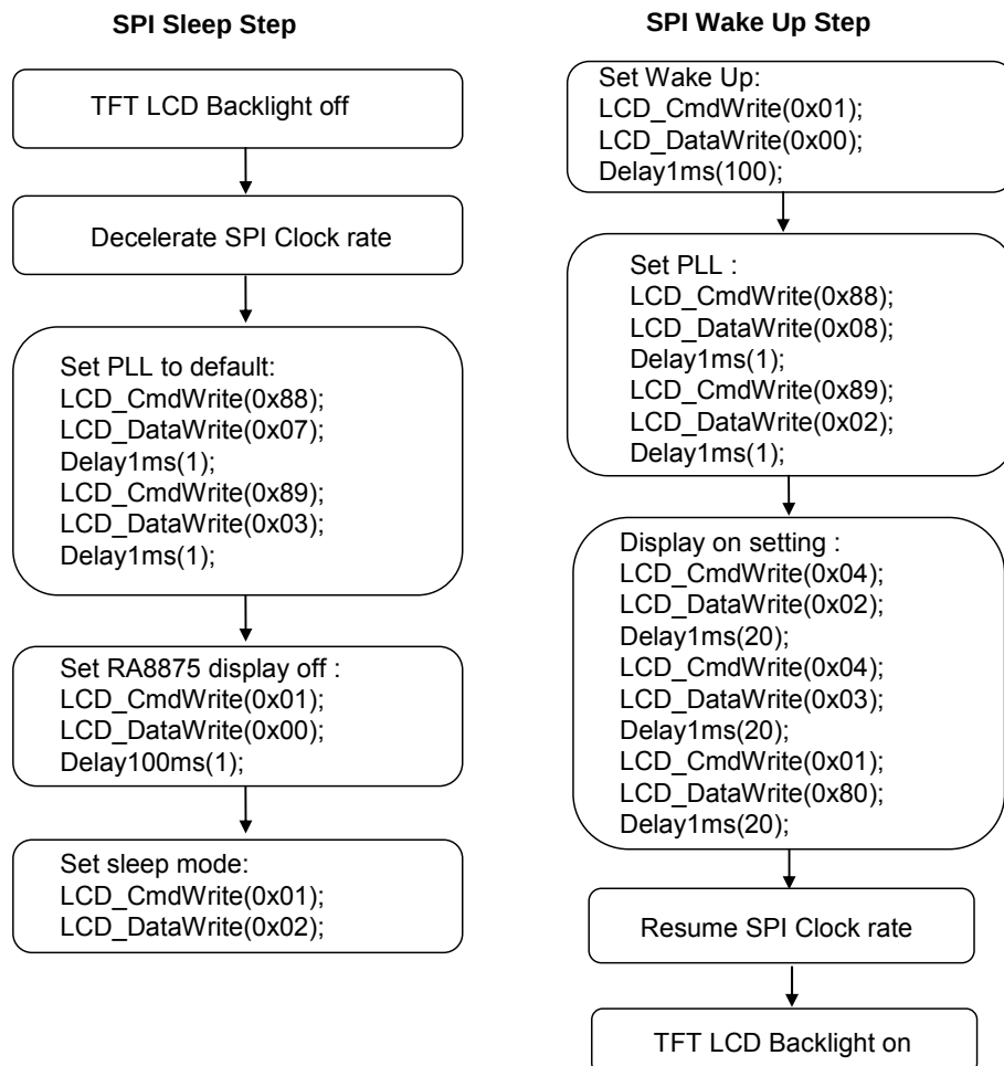
圖6-20 : SPI 睡眠/喚醒
