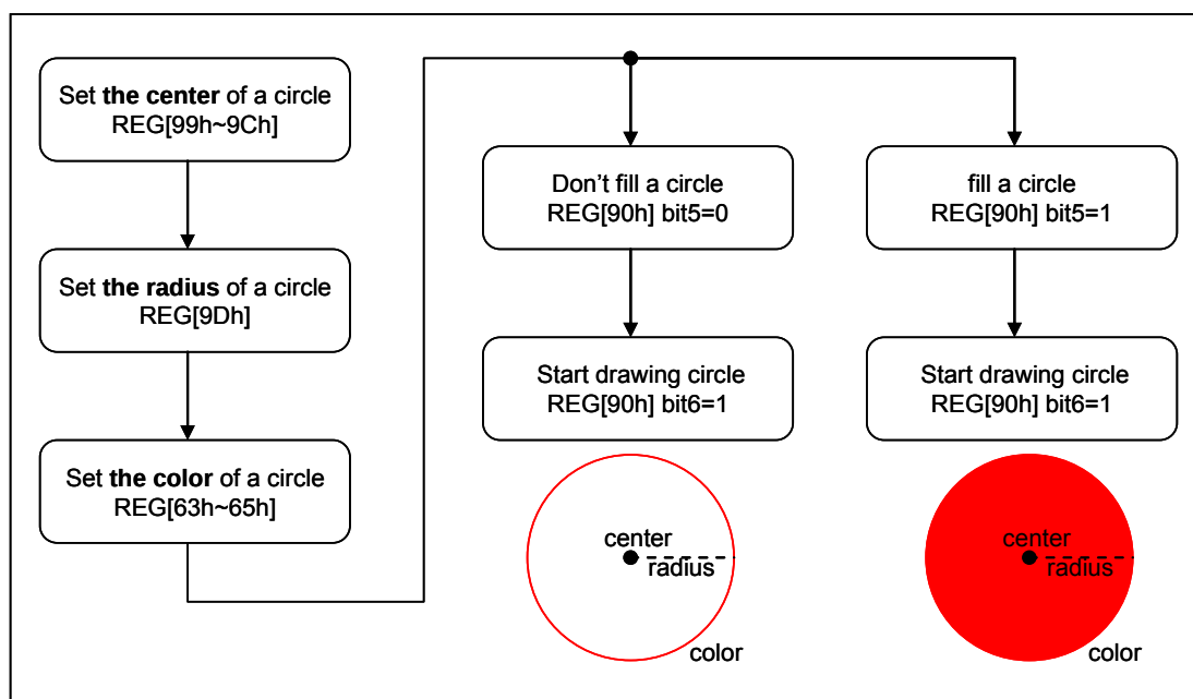
图 7-26 : 绘图功能 - 画圆
