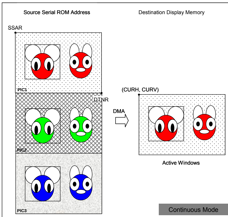
图 7-83 : 连续数据存储器存取模式
