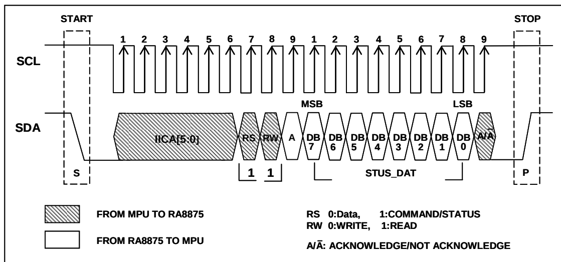
图 6-25 : 数据总线的状态读取
