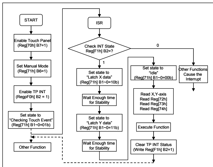
图 7-79 : 触控面板手动模式流程图
