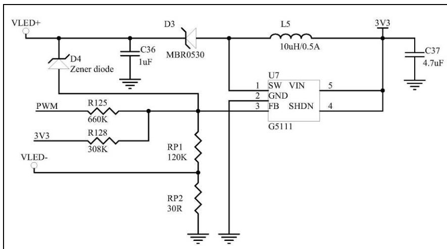
图 6-50 : PWM 控制 TFT 面板背光的应用电路
