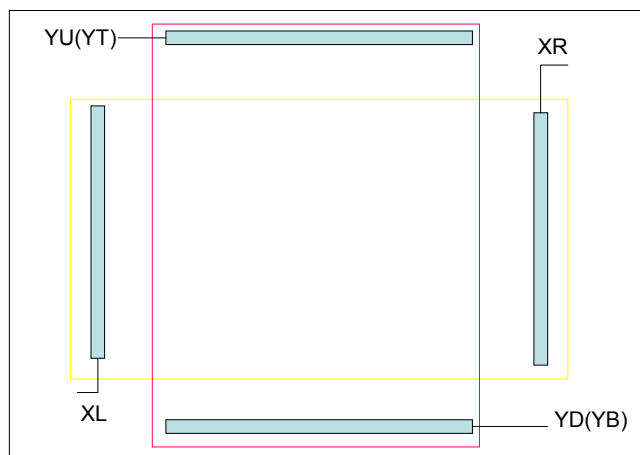
图 6-46 : 4-wire 触控面板架构
