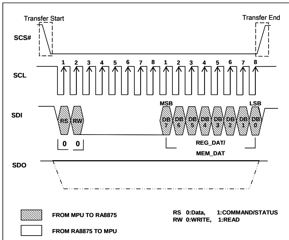
图 6-14 : 4-Wire SPI 数据总线的数据写入
