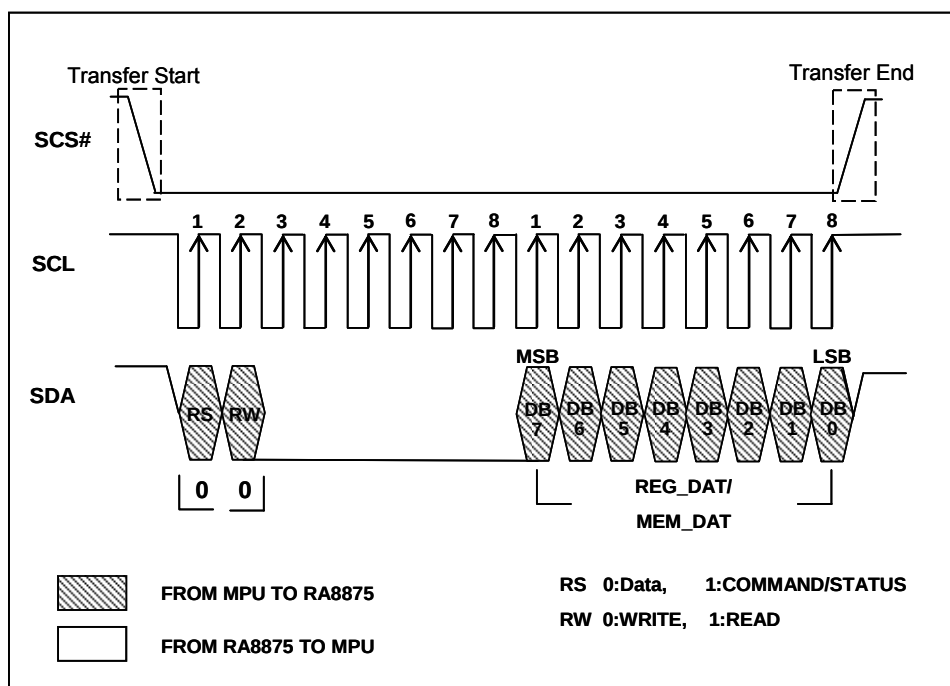
图 6-8 : 3-Wire SPI 数据总线的数据写入
