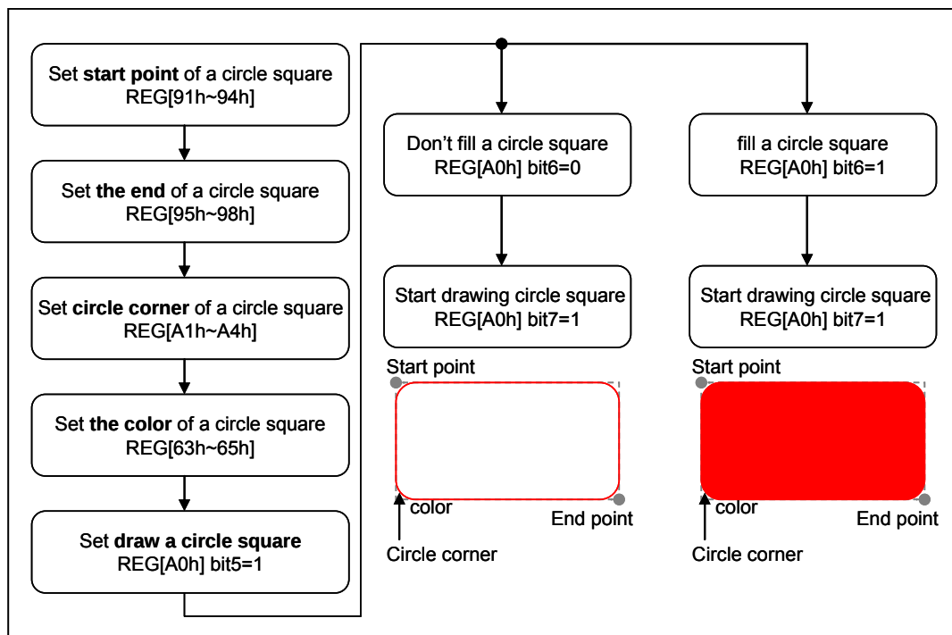
图 7-32：绘图功能 - 画圆角方型
