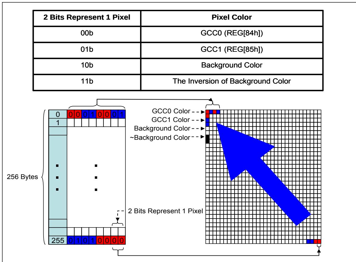
图 7-10 : 内存对应和图形光标的关联
