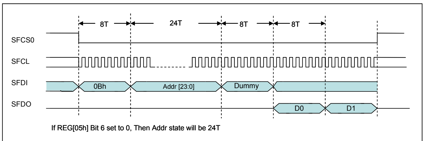
图 6-41 : 5-BUS (快速) 读取
