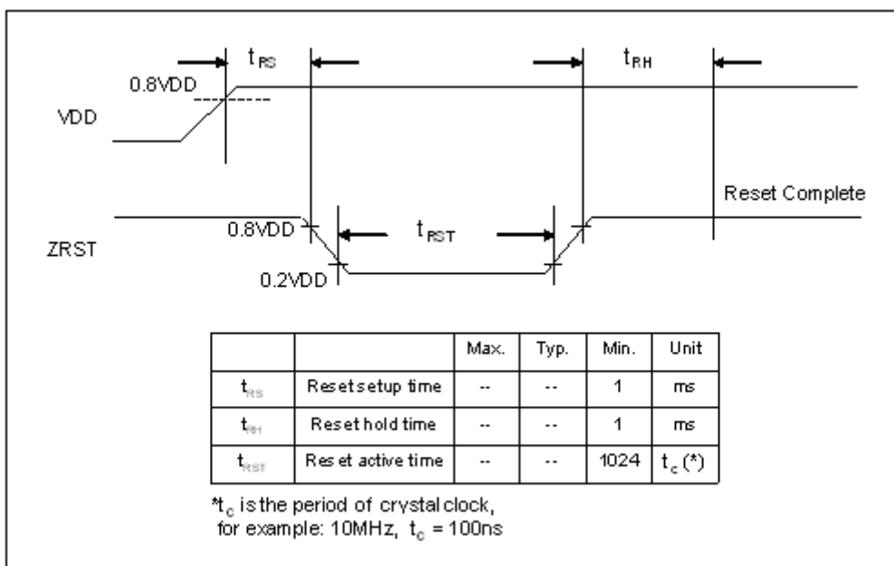
图 6-53 : 复位时序参数
