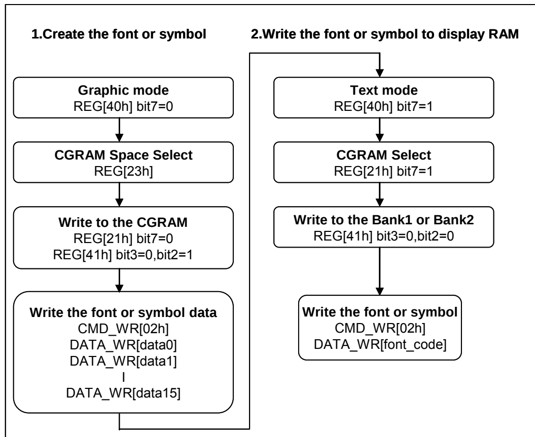
图 7-20 : CGRAM 的写入程序
