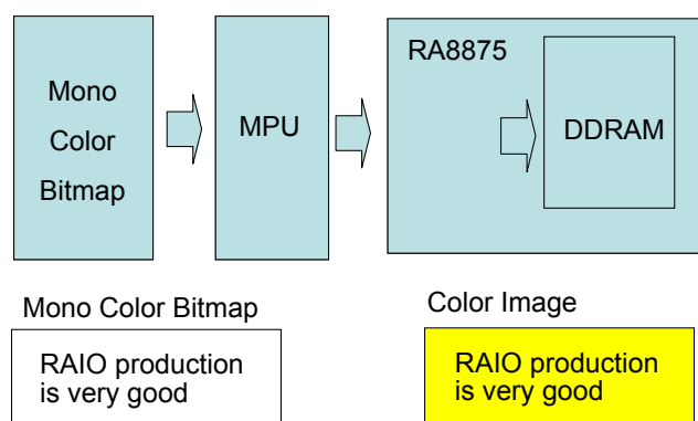
图 7-57 : 颜色扩充功能的数据区块图
