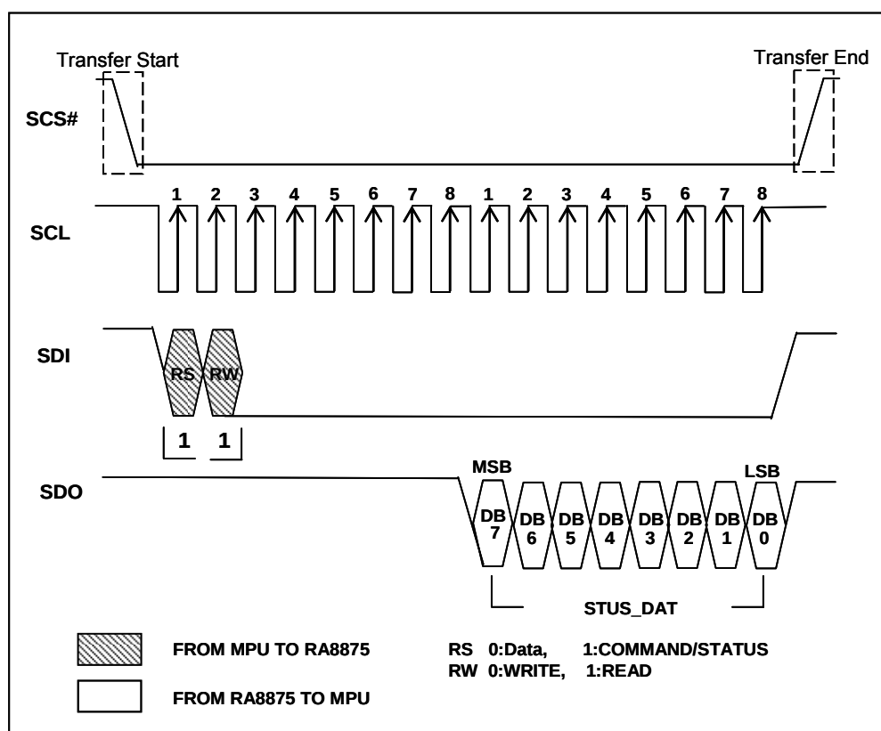
图 6-17 : 4-Wire SPI 数据总线的状态读取
