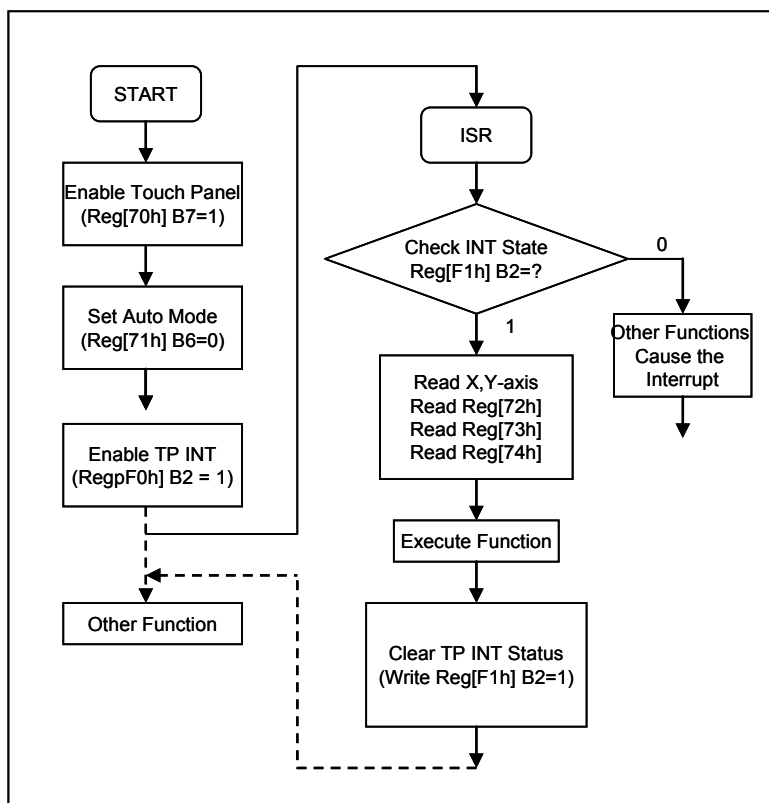
图 7-78 : 触控面板自动模式流程图
