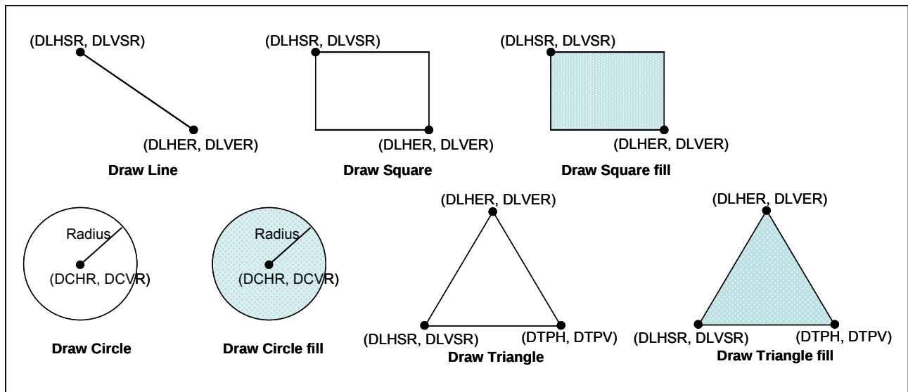
图 5-6 : 绘图功能参数
