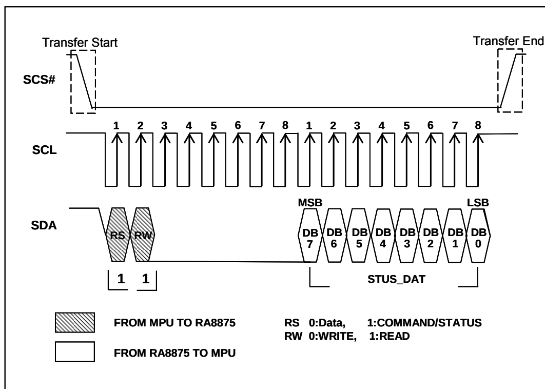
图 6-11 : 3-Wire SPI 数据总线的状态读取
