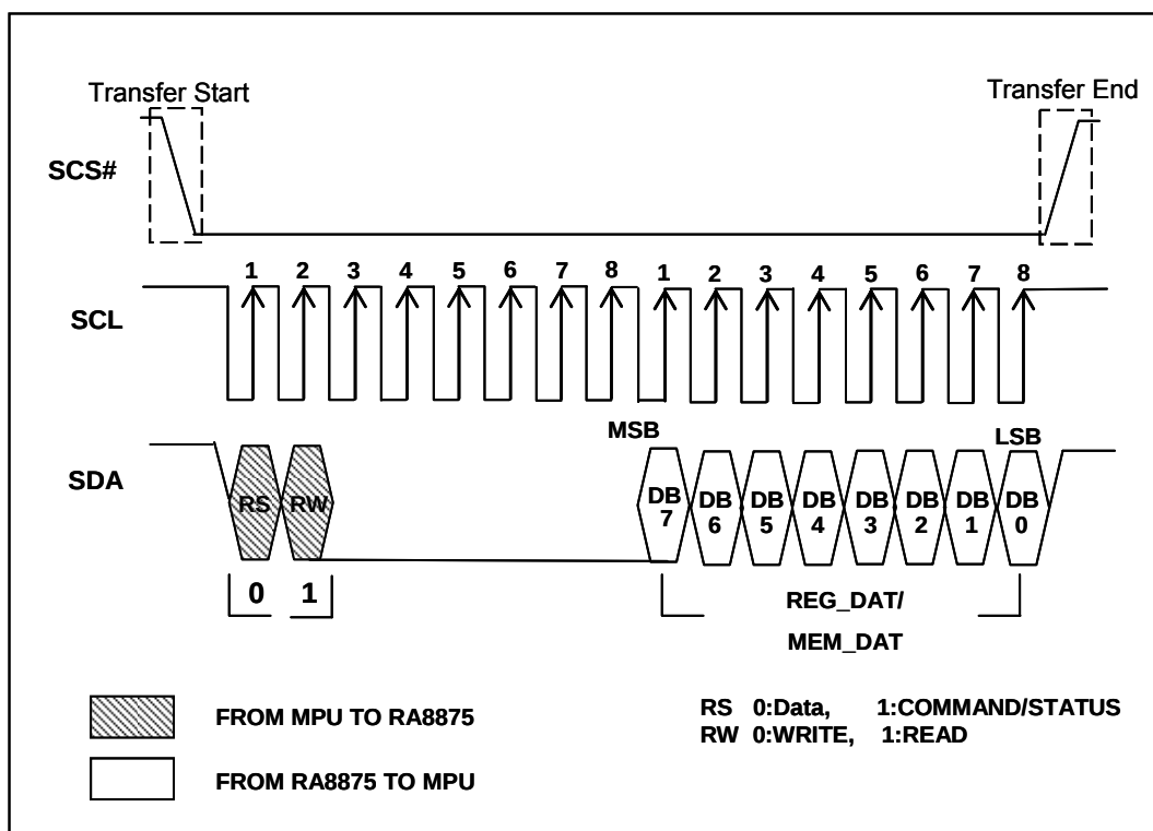
图 6-9 : 3-Wire SPI 数据总线的数据读取
