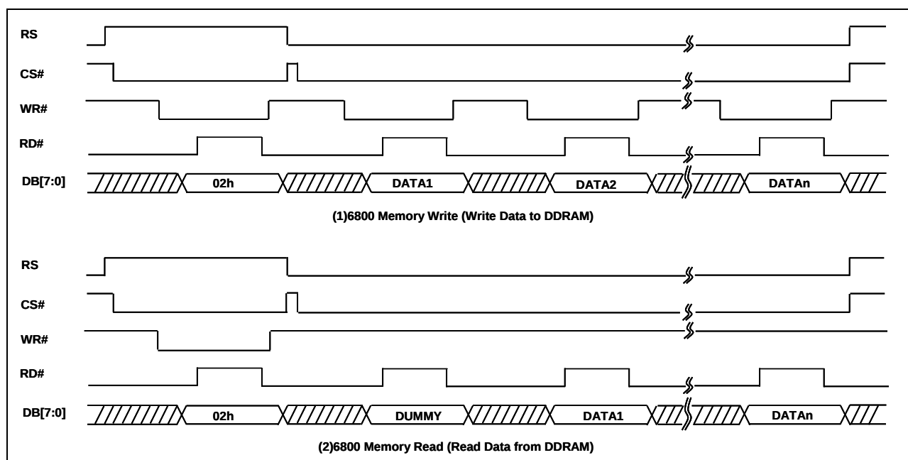
图 6-31 : 6800 内存写入与内存读取
