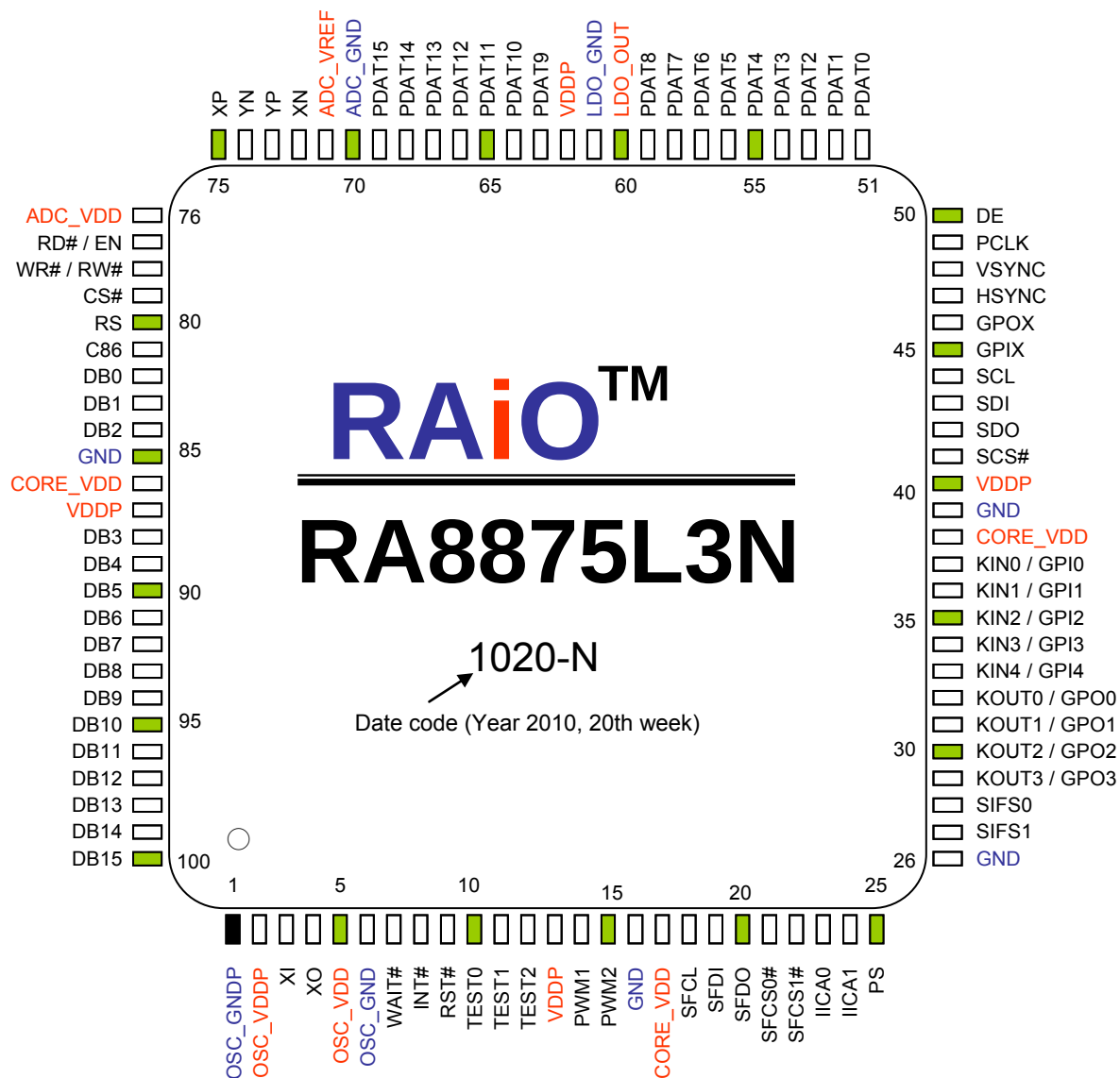
图 9-1 : RA8875 的接脚图
