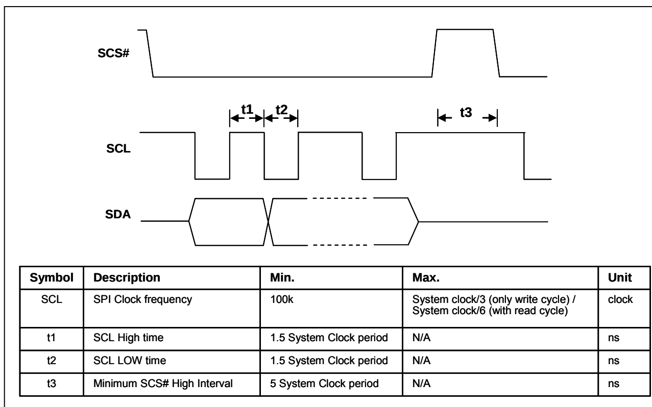
图 6-12 : 3-Wire 的 SPI 时序
