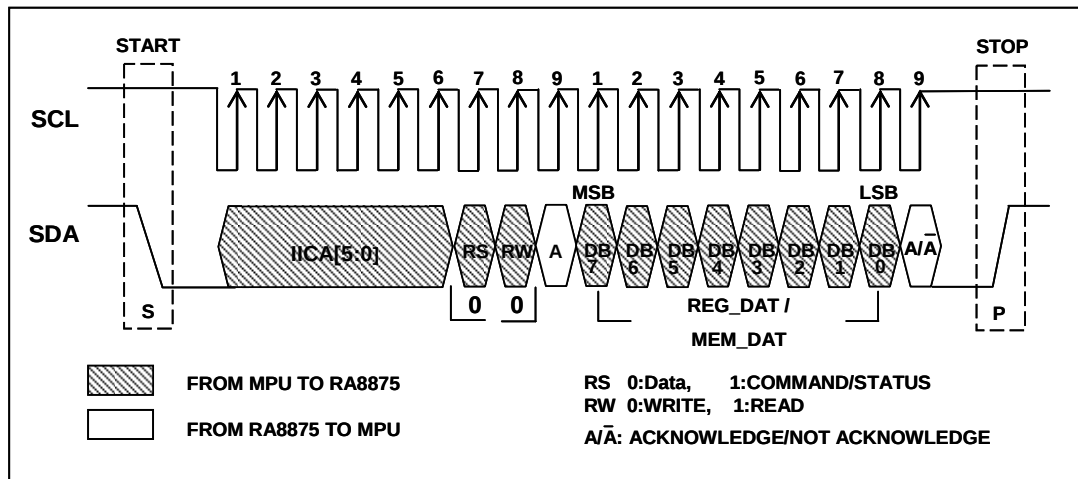
图 6-22 : IIC 数据总线的数据写入
