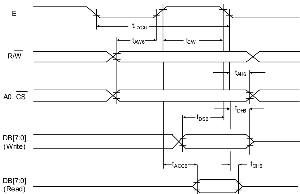
图 6-3 : 6800 MCU 传输协议
