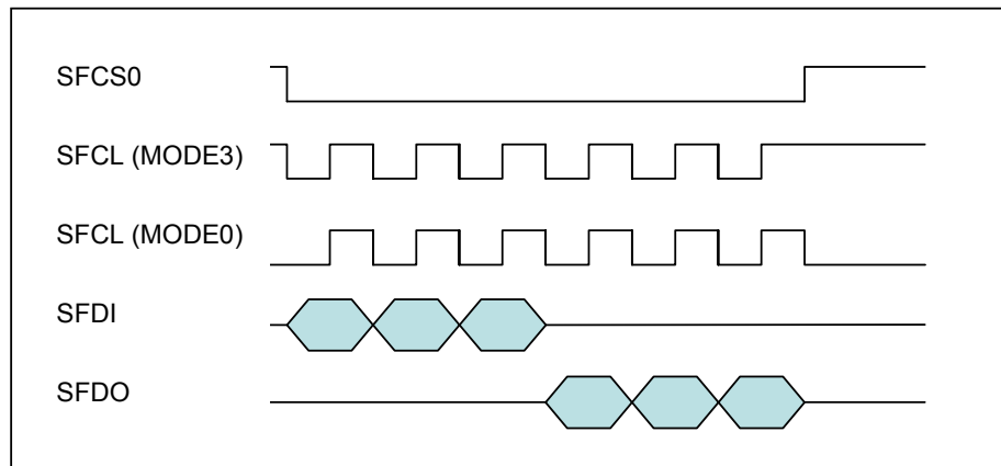
图 6-39 : Mode 0 与 Mode 3 的传输方式
