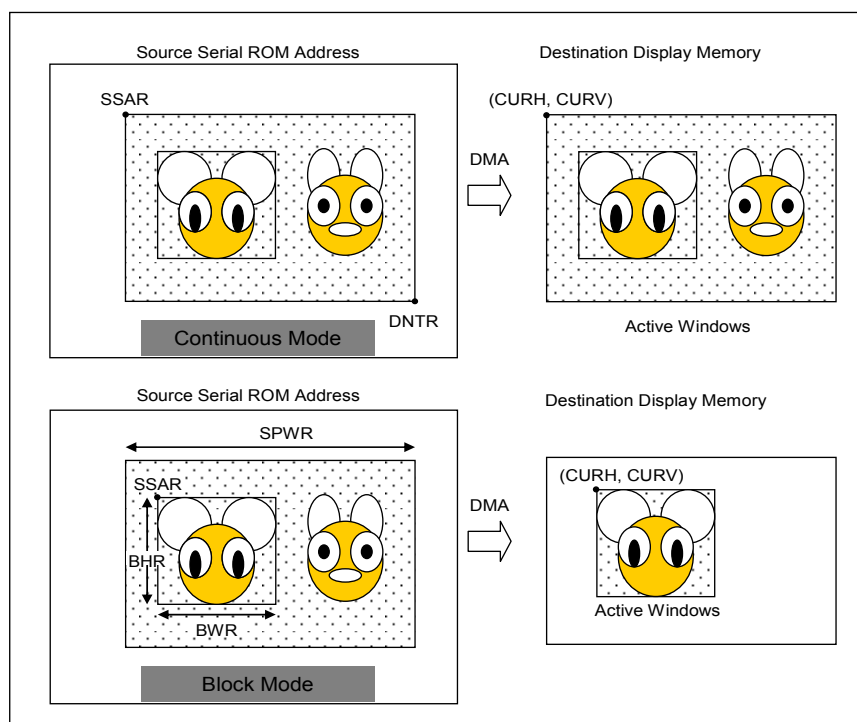
图 5-8 : DMA 连续性模式与区块模式
