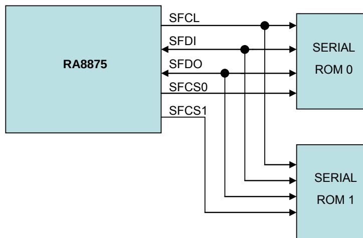
图 6-38 : RA8875 串行式 Flash/ROM 系统
