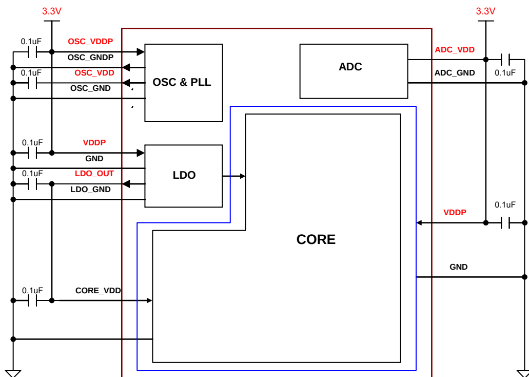
图 6-54 : RA8875 的电源接法
