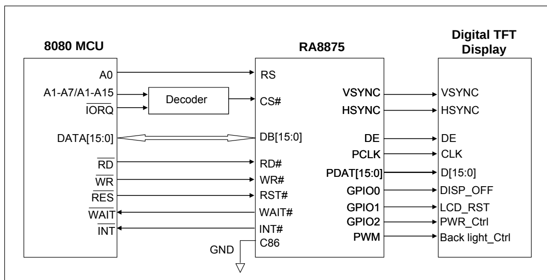
图 6-37 : RA8875 与数位 TFT 界面
