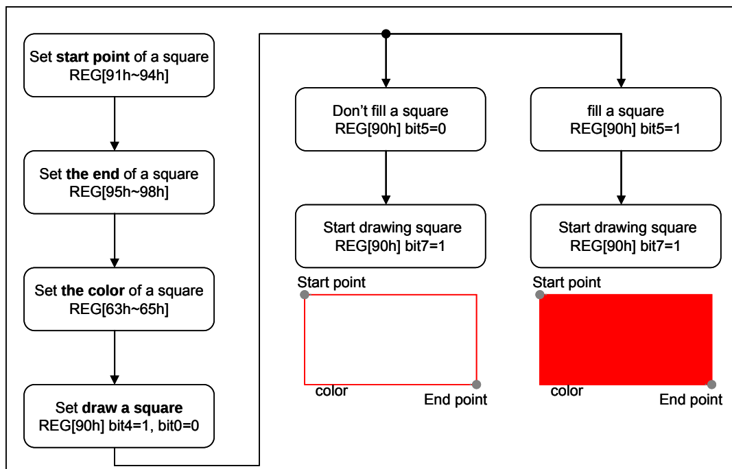
图7-29 : 绘图功能 - 画方形
