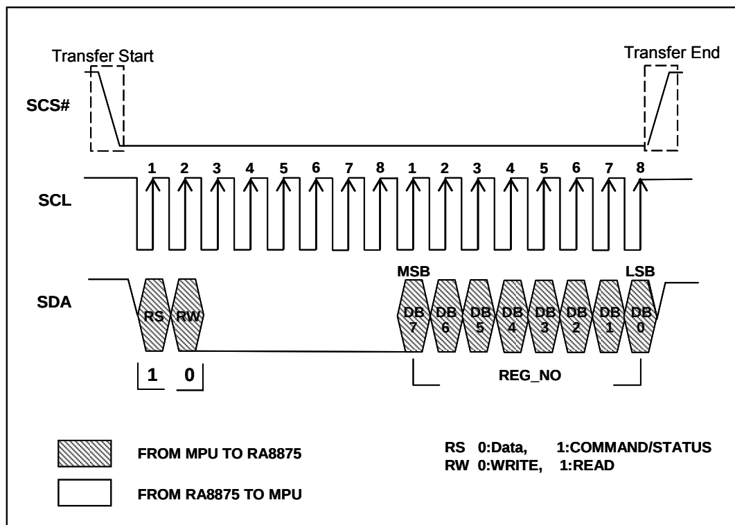
图 6-10 : 3-Wire SPI 数据总线的指令写入
