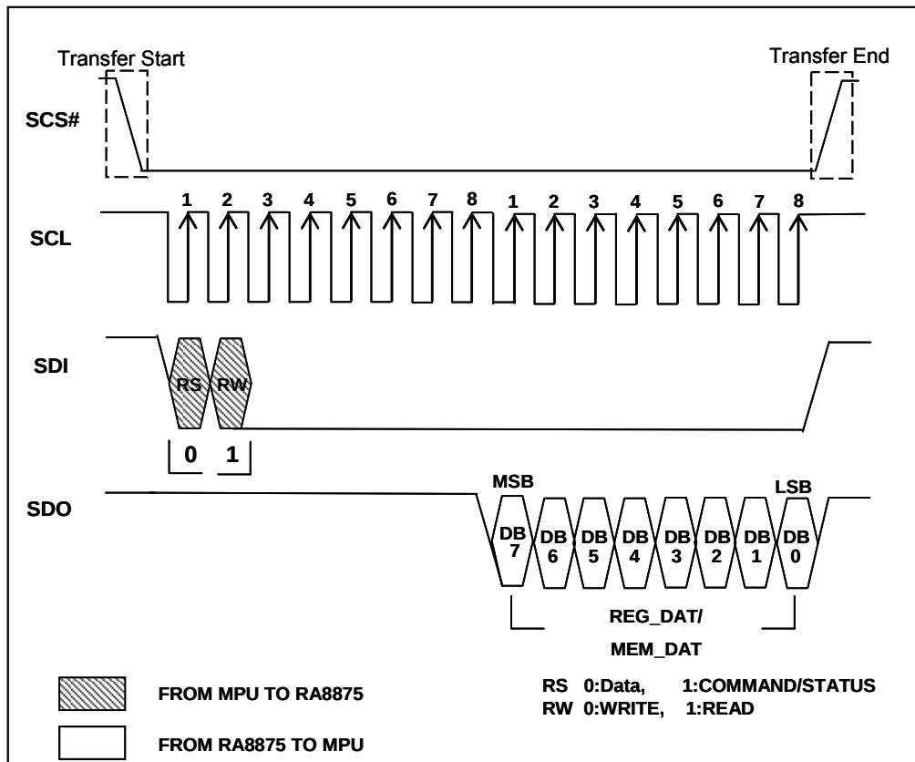
图 6-15 : 4-Wire SPI 数据总线的数据读取
