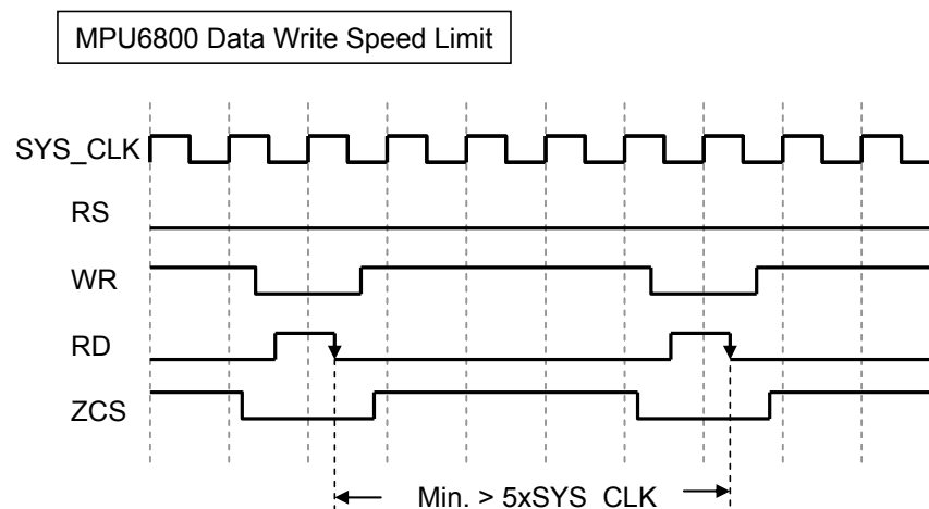
图 6-5 : 6800 接口连续性数据写入周期图
