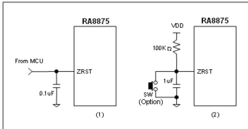
图 6-52 : RST# 接脚的使用范例
