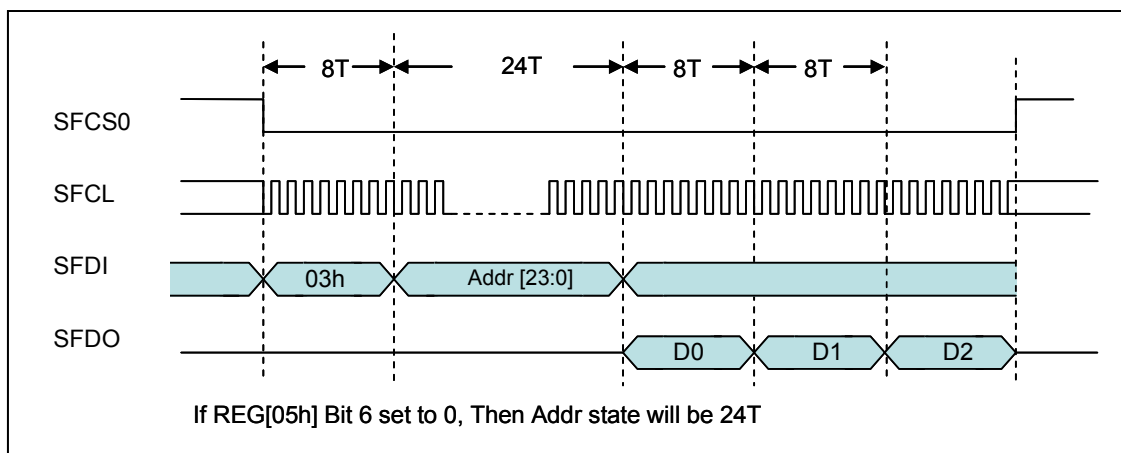
图 6-40 : 4-BUS (正常) 读取
