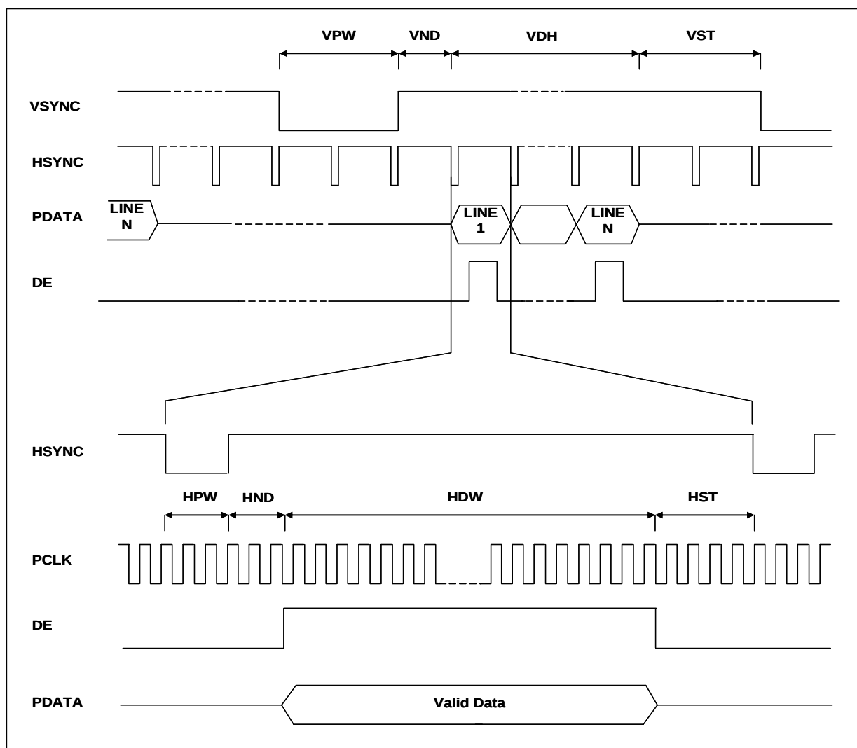
图 6-36 : 数位 TFT 面板时序图
