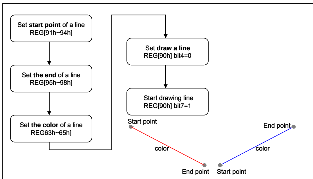
图 7-30 : 绘图功能 - 画直线
