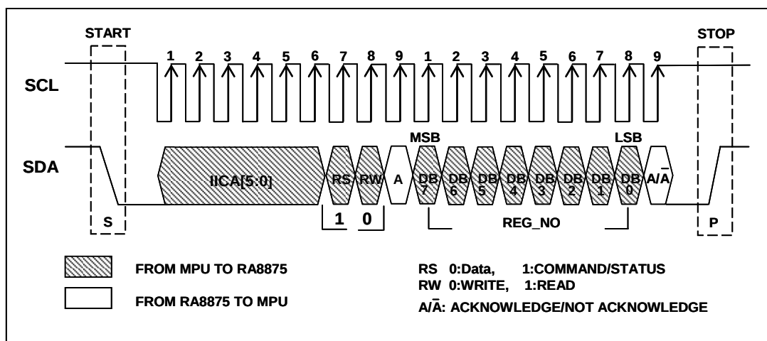
图 6-24 : IIC 数据总线的指令写入
