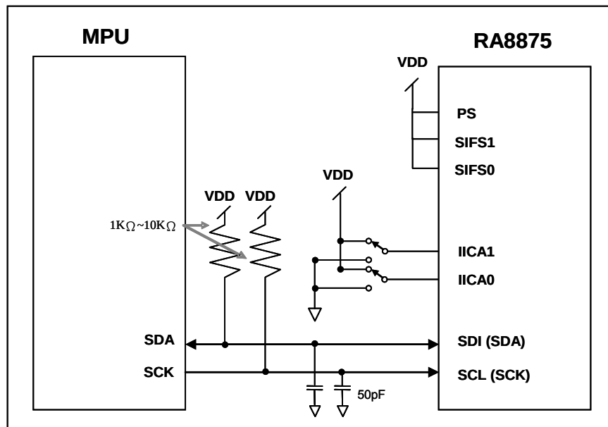
图 6-21 : IIC 的 MCU 界面图
