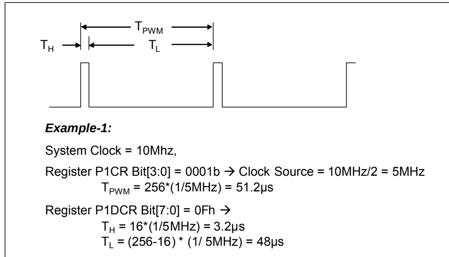
图 7-86 : PWM 输出脉冲范例二
