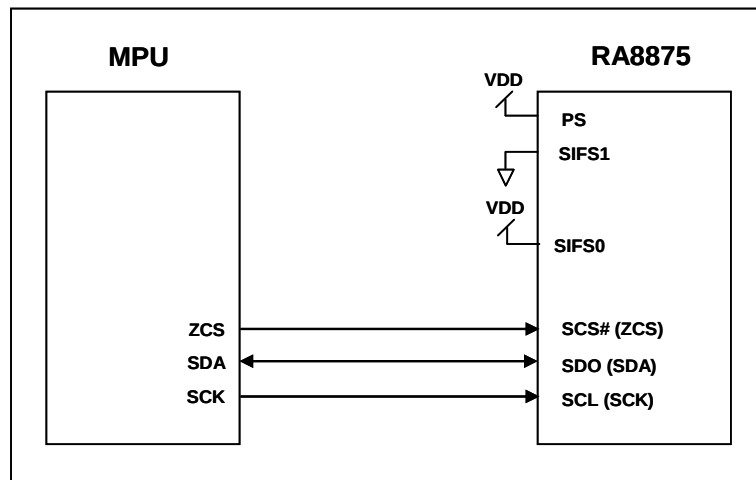
图 6-7 : 3-Wire SPI 的 MCU 界面图
