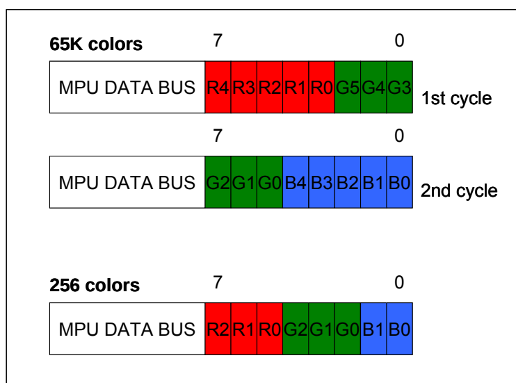
图 6-34 : MCU 8-bit 时 Data Bus 所对应到的 RGB 数据
