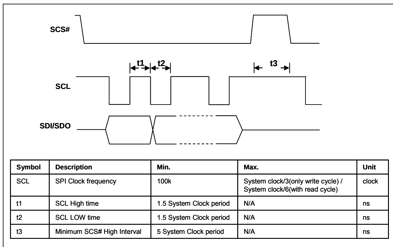
图 6-18 : 4-Wire 的 SPI 时序
