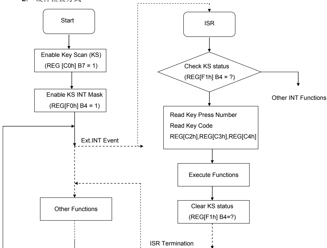
图 7-81：键盘扫描流程图 _ 硬件中断
