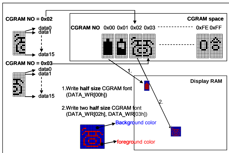
图 7-21 : CGRAM 的写入图示
