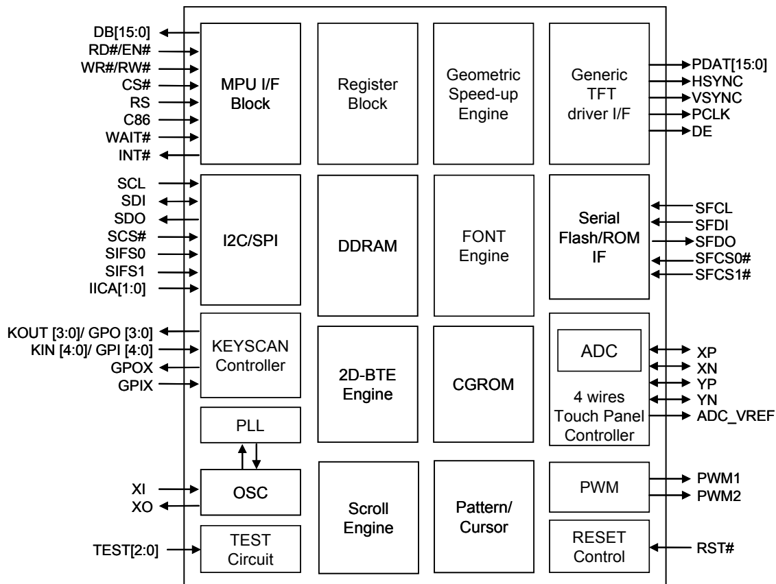
图 3-1 : RA8875 内部方块图
