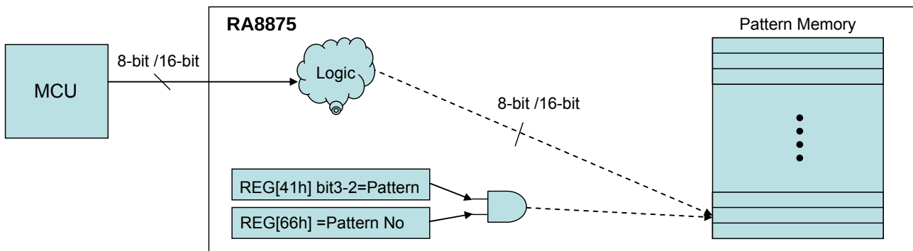
图 7-17 : 8/16 位的色彩模式
