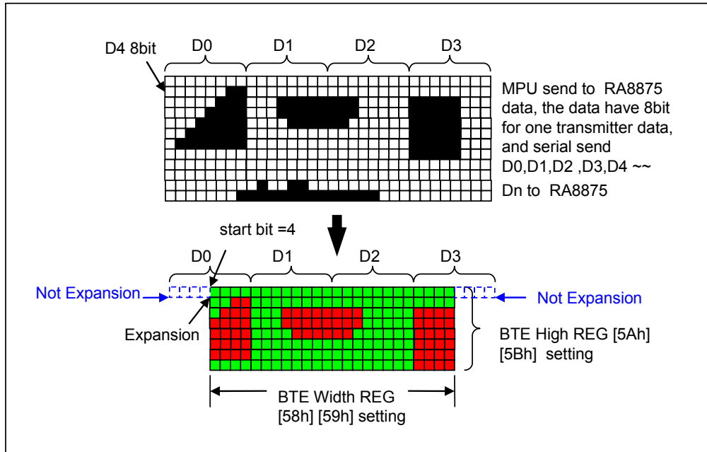
图 7-60 : 颜色扩充功能数据示意图
