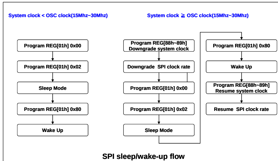
图 6-19 : SPI 睡眠/唤醒流程
