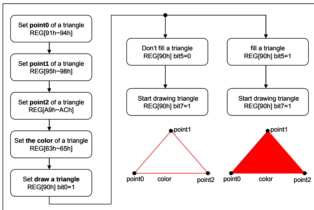
图 7-31 : 绘图功能 - 画三角形
