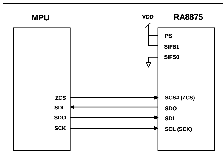
图 6-13 : 4-Wire SPI MCU 界面图
