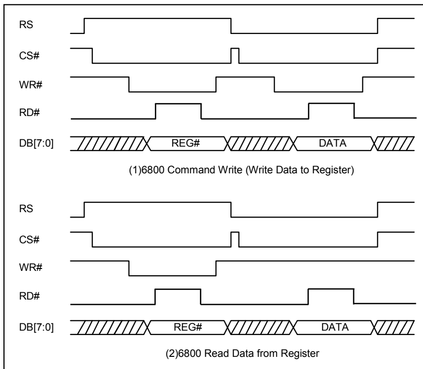
图 6-29 : 6800 「指令写入到寄存器」与「寄存器读取」
