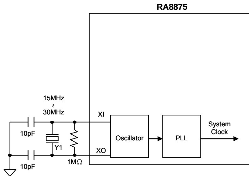
图 6-51：石英震荡电路与系统频率的产生
