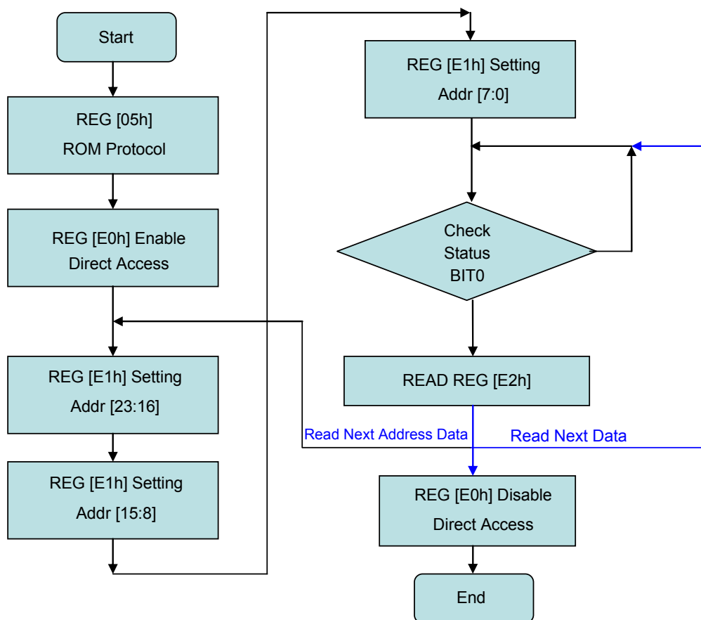
图 6-45 : 直接存取模式流程图
