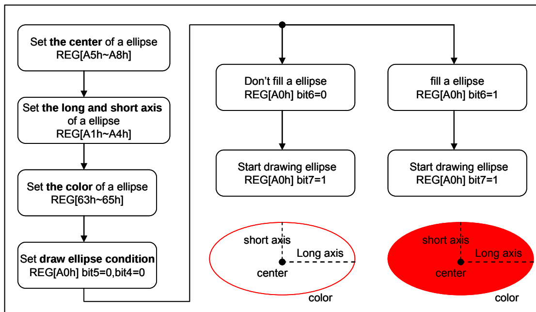
图 7-27 : 绘图功能 - 画椭圆
