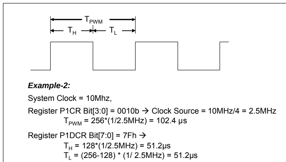
图 7-85 : PWM 输出脉冲范例一
