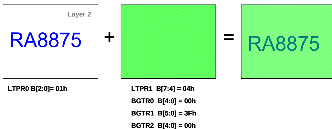
图 7-71 : 图层二与通透模式的显示效果
