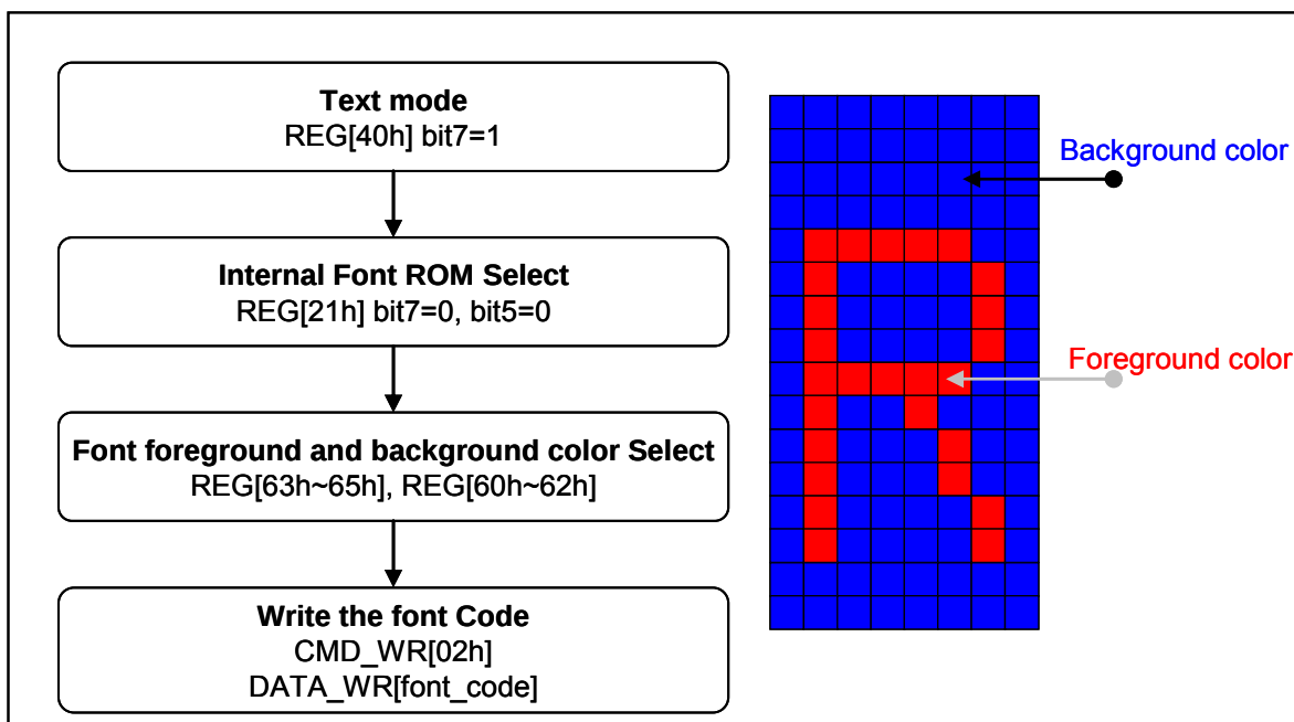
图 7-18 : ASCII 字型 ROM 的写入程序
