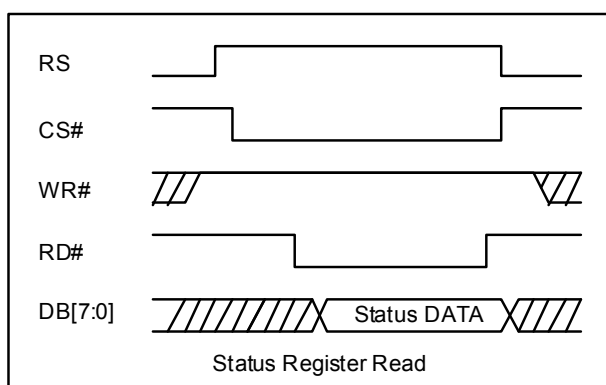
图 6-26 : 8080 状态读取寄存器
