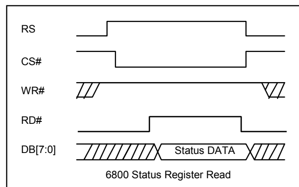
图 6-27 : 6800 状态读取寄存器
