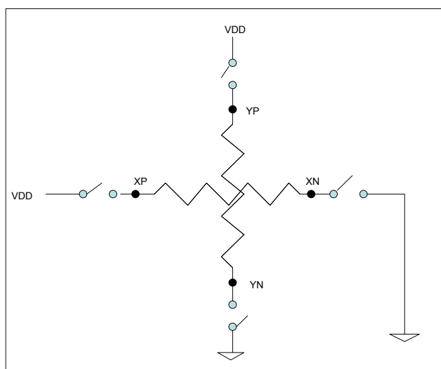
图 6-47 : 4-wire 触控面板原理
