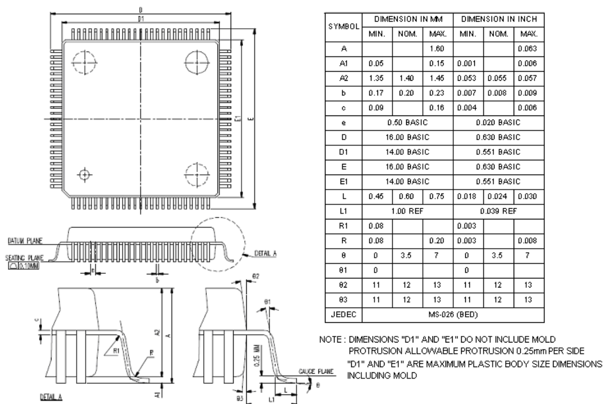
图 9-2 : RA8875 的外观尺寸
