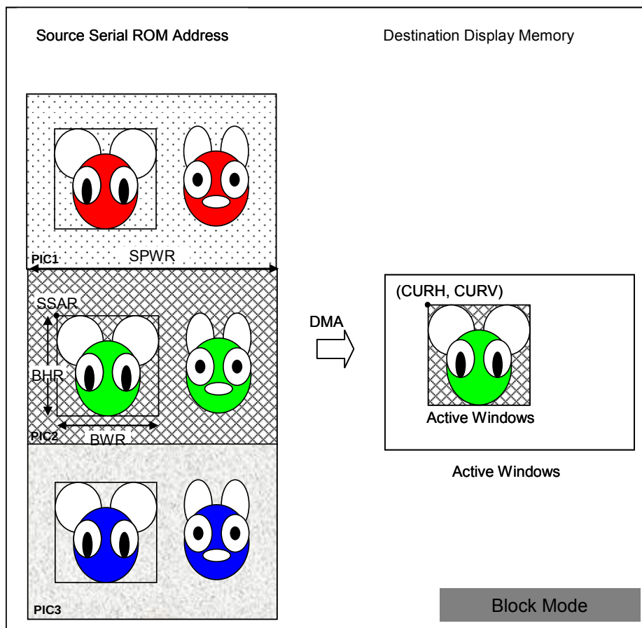
图 7-84：区块数据存储器直接存取模式
