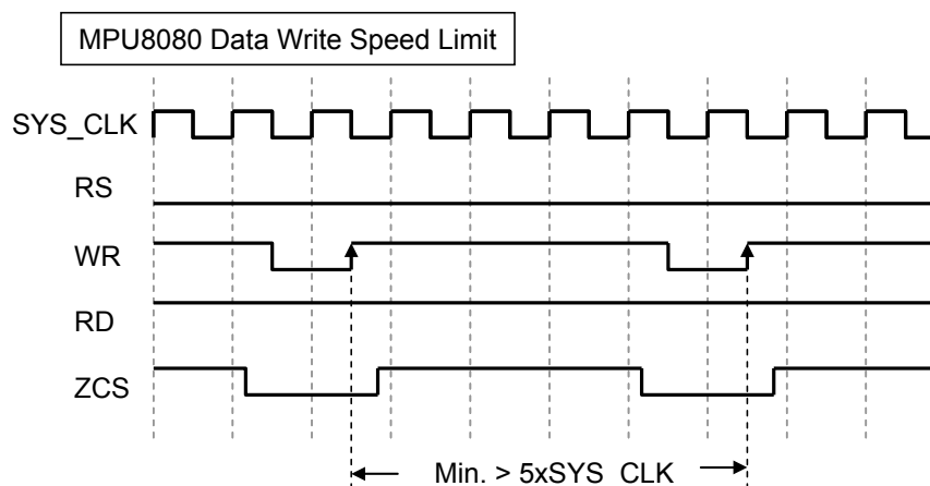
图 6-6 : 8080 接口连续性数据写入周期图
