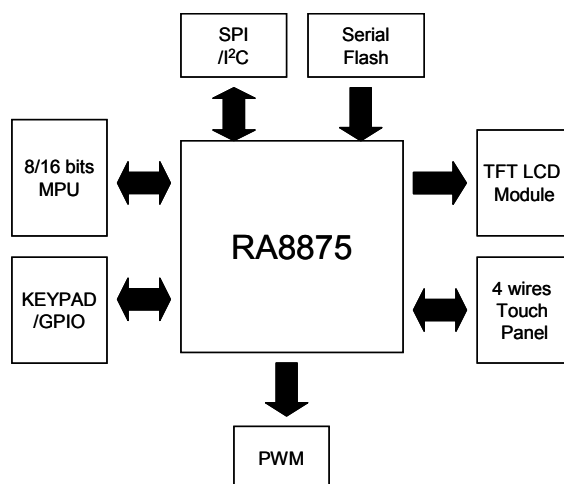
图 3-2 : RA8875 系统方块图
