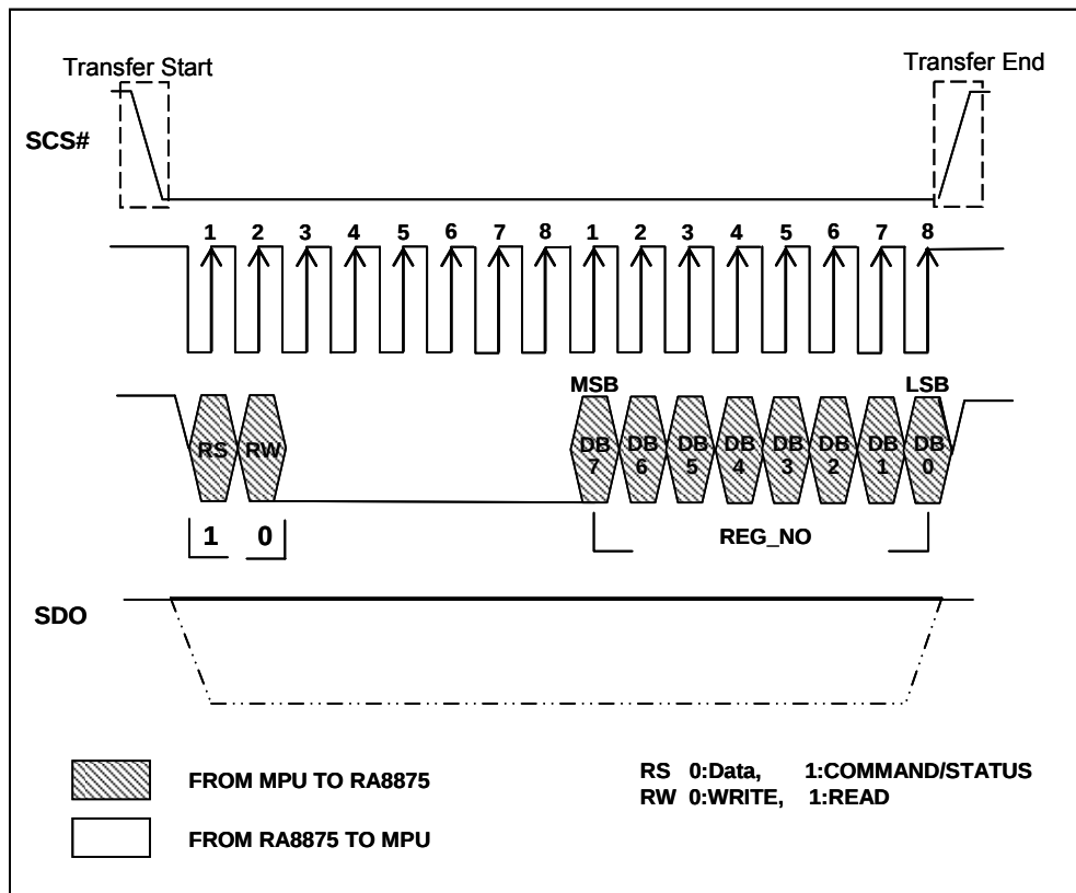
图 6-16 : 4-Wire SPI 数据总线的指令写入
