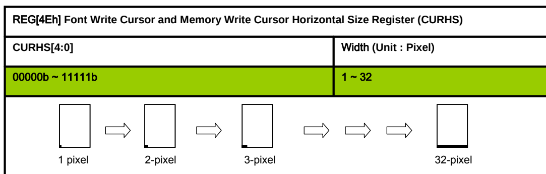
图 7-14 : 记忆体写入时光标宽度设定
