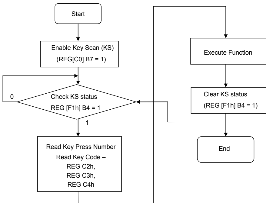
图 7-80：键盘扫描功能的流程图 _ 软件轮询
